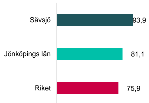
Figur 14 - Demografisk försörjningskvot, 2018
